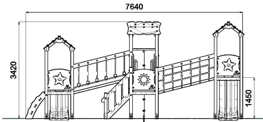
VISTA LATERALE
