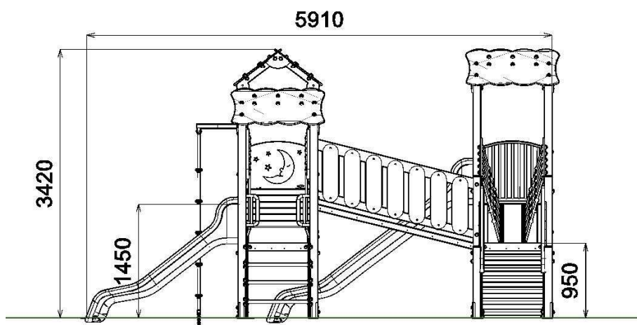
VISTA LATERALE
